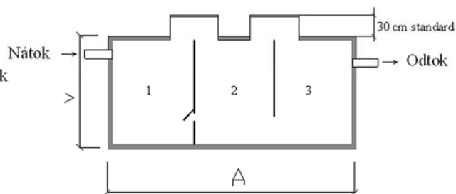
SEPTIK PPSH
